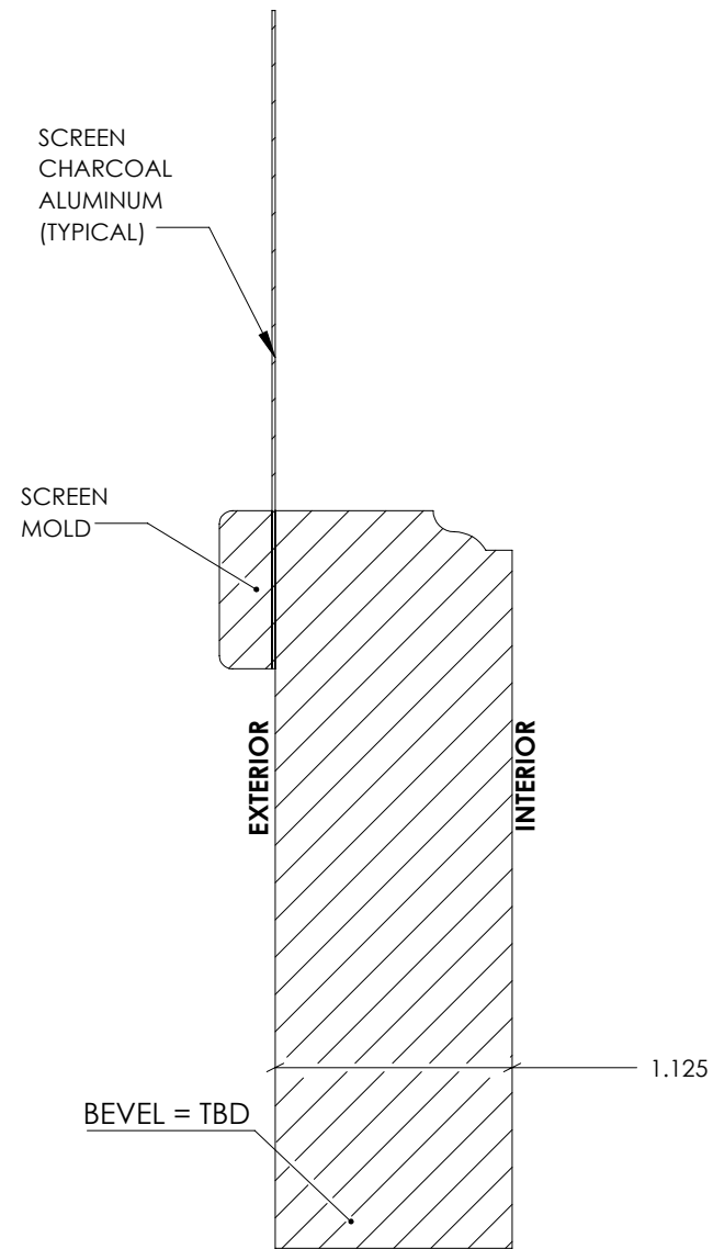
SECTION A-A
